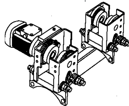
afbeelding 3-3 monoraalkat
