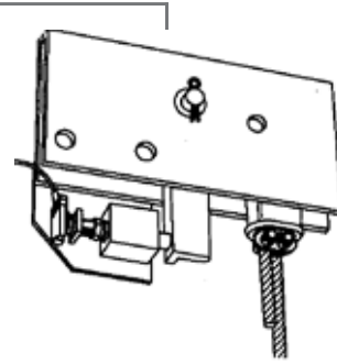
afbeelding 2-5 overlastbeveiliging
