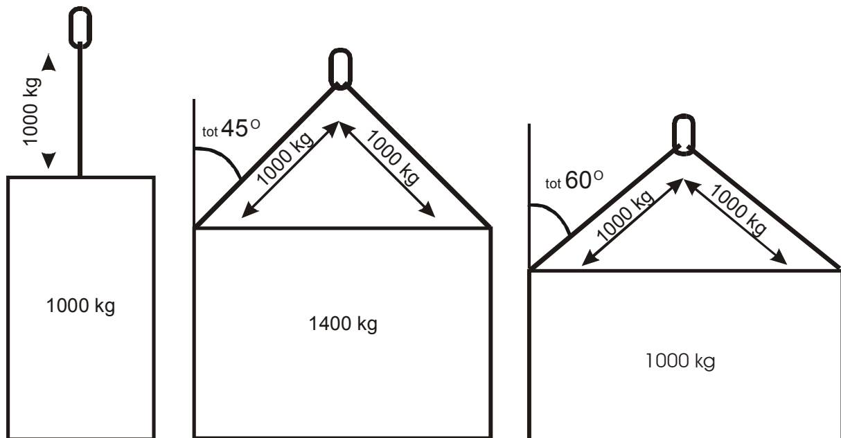
afbeelding 5-16 optredende krachten (1)
