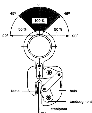
afbeelding 4-26 vloerenklem
